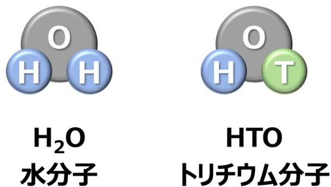
図 2. 水分子とトリチウム水の違い.
